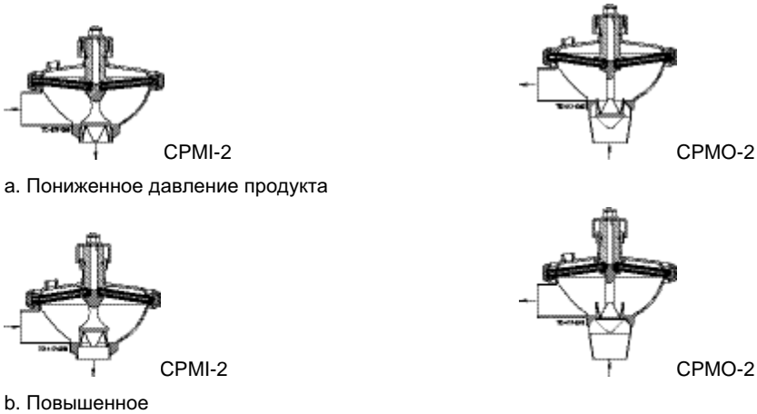
Рис. 3. Принцип действия клапанов
