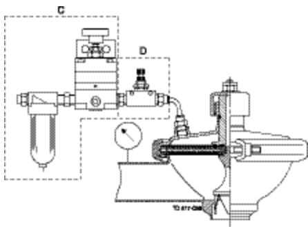
Рис. 5. Клапан СРМІ-2 с клапаном для регулирования давления сжатого воздуха и манометром.
