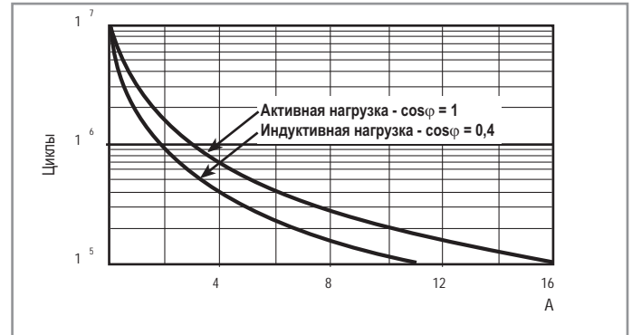
F 46 – График зависимости электрического ресурса при нагрузке АС от тока нагрузки Тип 46.61
