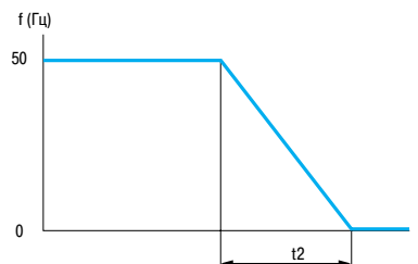
Линейная кривая торможения
